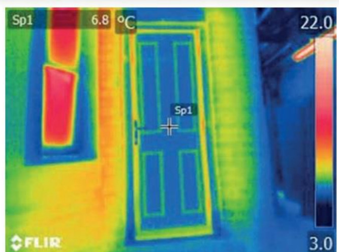
Consort GRP composite door
